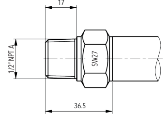
8845.XX.XX39.XX.XX.XX > 25 bar
