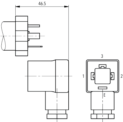
8845.XX.XXXX.05.XX.58
