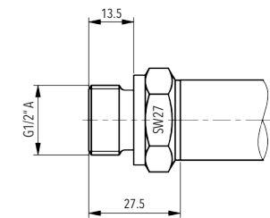
8845.XX.XX21.XX.XX.XX ≤ 25 bar
