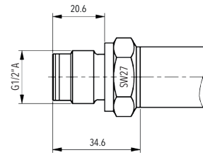
8845.XX.XX31.XX.XX.XX
