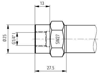
8845.XX.XX10.XX.XX.XX ≤ 25 bar
